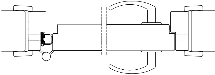
Infällt klämskydd : brandklass upp till E30/EI30 och ljudreduktion upp till 38 dB
